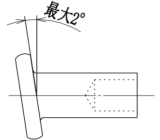
座面の傾き
